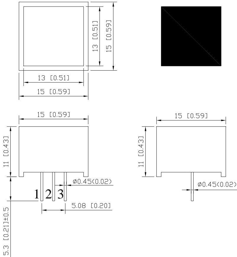
KWL-R154AVW
